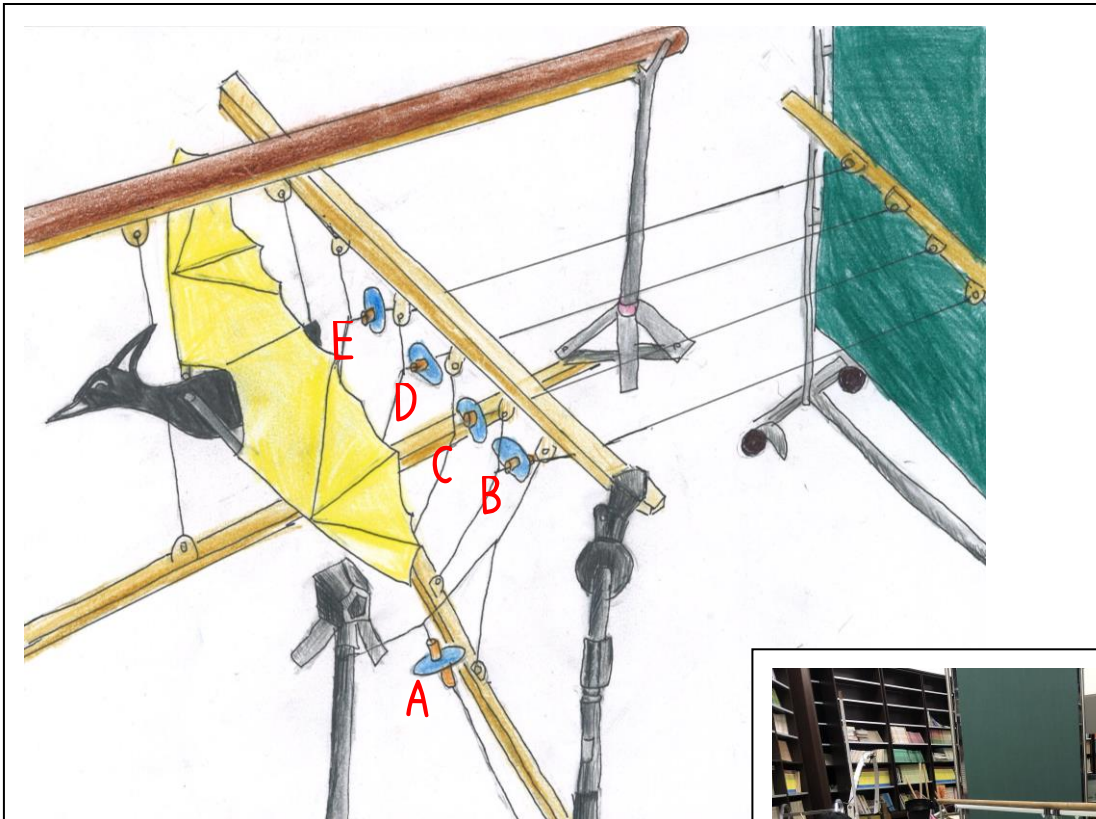
圖 6-10：將 5 個「氣流流速測試儀」分別置於撲翅機的側面及平均分布於翅膀後方，並依區域命名為 A、B、C、D、E。
