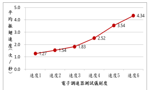
圖 8-4：撲翅機刻度與振翅速度關係圖
