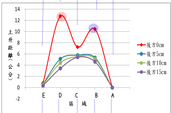
圖 7-6：振翅速度 4.34 次/秒，上方 5cm，各區域「氣流流向測試儀」距機身遠近與其上升距離關係圖
