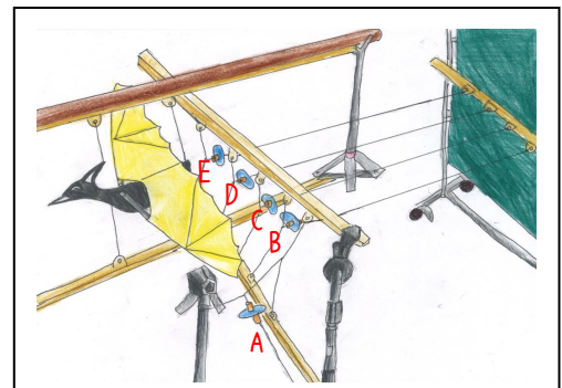
圖 8-8：將「氣流流向測試儀」水平架設則可量測水平氣流。
