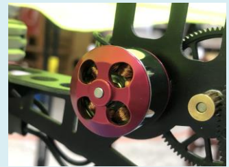
圖 2-4：選用散熱佳、重量輕、馬力大的遙控直升機專用之 KV3800 型號高速馬達。
