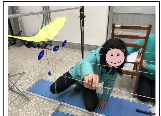
圖 6-12：利用棉繩上的尺規記號計數「氣流流向測試儀」的移動距離。
