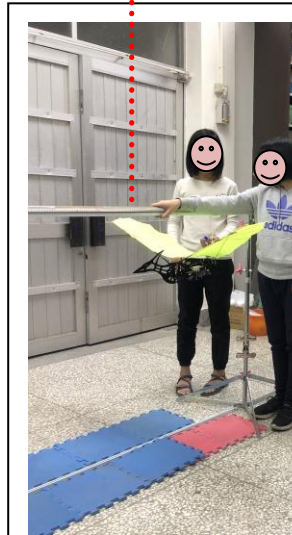
圖 2-9：實驗環境布置。
