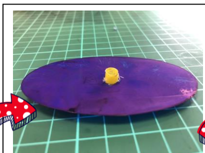
圖 6-6：「氣流流向測試儀」本體完成囉！
