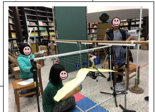
圖 6-11：實驗環境實景照
