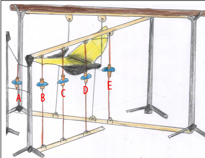
圖 7-1：將 5 個「氣流流向測試儀」分別置於「撲翅機」側面及平均分布於翅膀後方，並依區域命名為 A、B、C、D、E。
