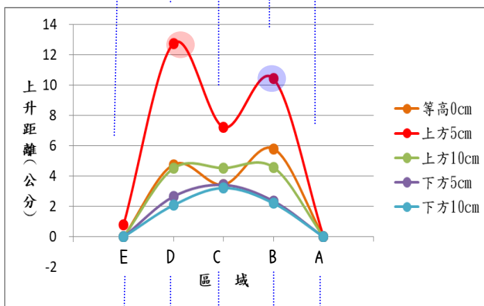
圖 7-5：「撲翅機」振翅速度 4.34 次/秒下，各區域「氣流流向測試儀」高度與其上升距離關係圖。
