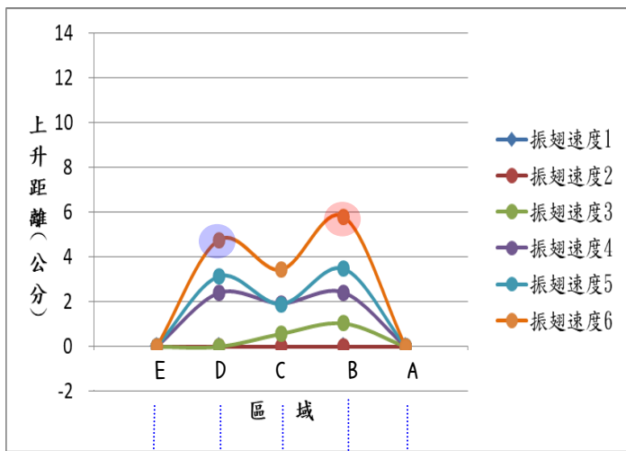
圖 7-4：6 種不同振翅速度與其各區域「氣流流向測試儀」上升距離之關係圖
