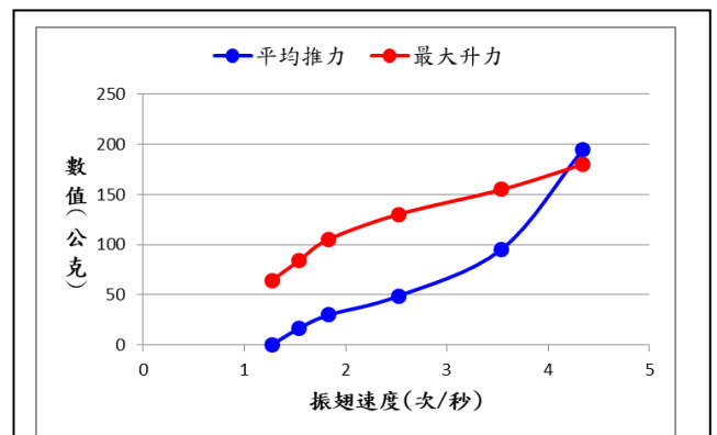
圖 8-5：撲翅機不同振翅速度下，其平均推力及最大升力關係圖。
